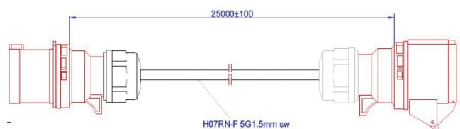
CEE 16A 5polig Stecker
